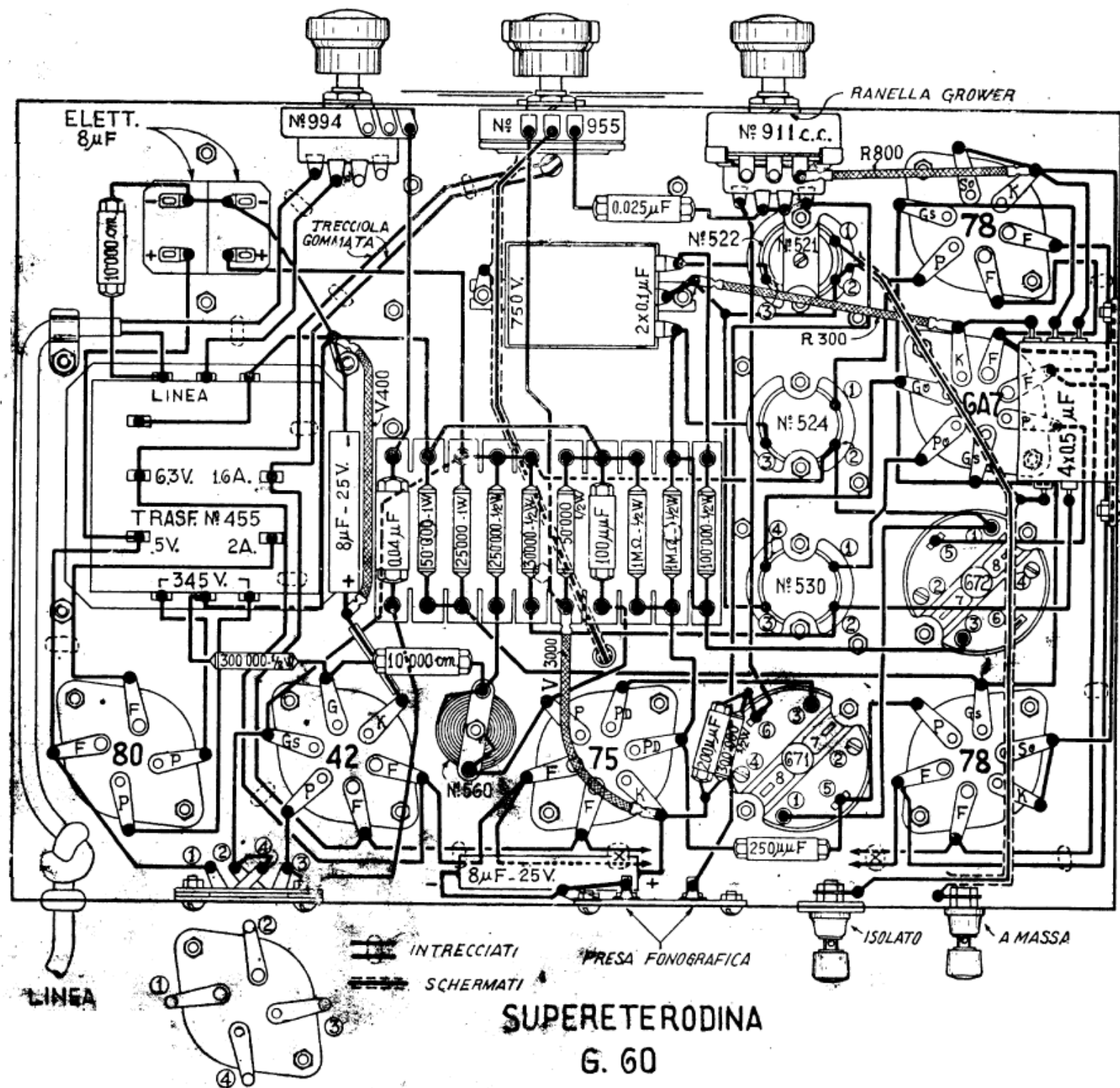
Schema elettrico della Super G-60.
